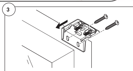
3 Outside window frame / Utsida vinduskarm / Utsida fönsterkarm / Karmin / Aknaraami külge
