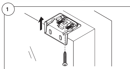
1 Inside window frame / Innsida vinduskarm / Innsida fönsterkarm / Karmin sisään / Aknaraami sisene
