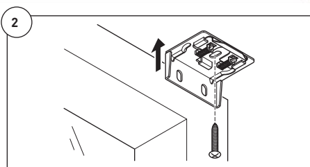
2 Ceiling mounting / Takfeste / Takfäste / Kattoasennus / Laekinnitus
